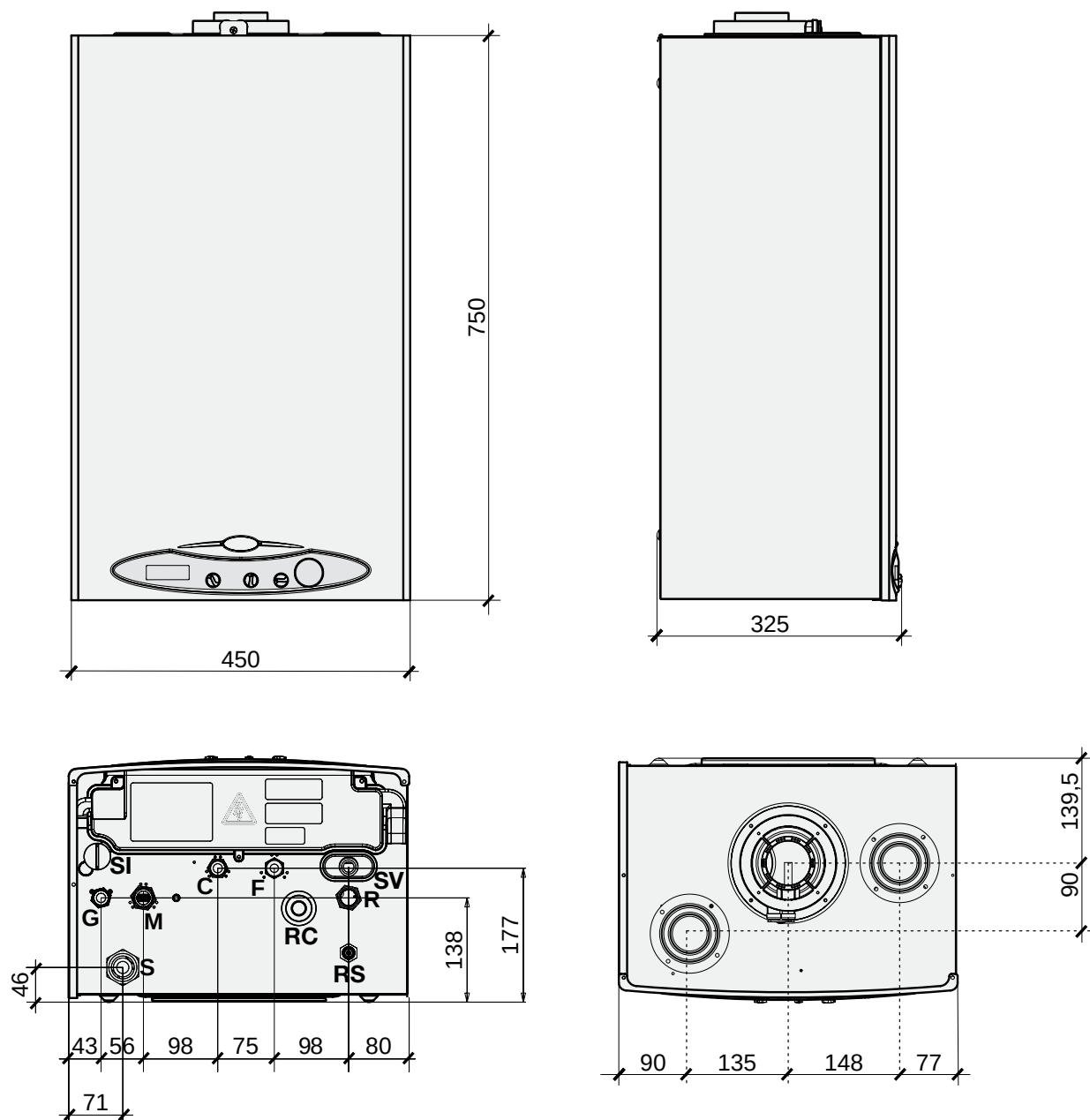
Vista dal basso modelli KC e KR
